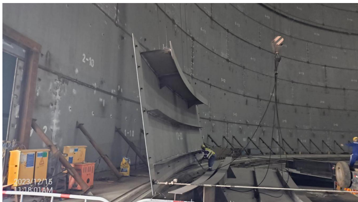
公示四：D#储罐第十二层内罐壁板安装照片
